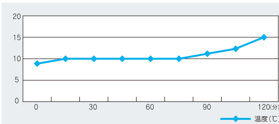
例 ショートケーキを入れた サービス箱 6号サイズでの保冷テスト
